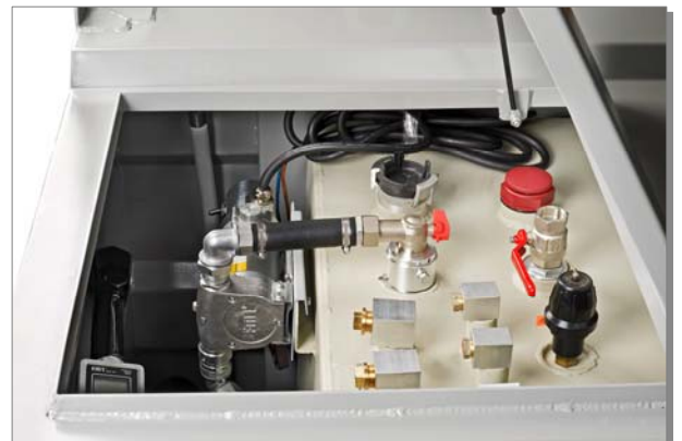
Cuve équipée d'une pompe
